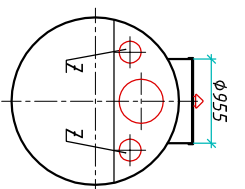
Разрез 2-2
